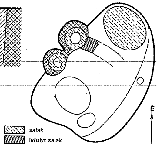
Nyugatmagyarországi vasolvasztó műhely alaprajza, XI-XII. sz. Nováki Gy. után
