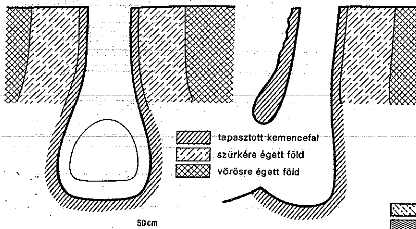
Imolai típusú buca-kemence metszete, Nováki Gy. után 40 Vastermelés és feldolgozás 900 és 1240 között
